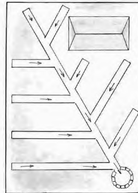
Рис. 1 Схема дренажа «ёлочки». Центральная дрена введена в дренажный колодец
